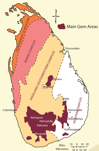
斯里兰卡主要宝石矿区域简化地图 (Gunaratne and Dissanayake, 1955年后)
